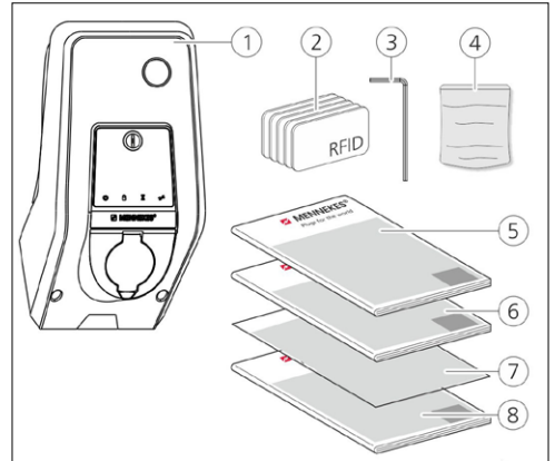
Abb.: 1. Lieferumfang
